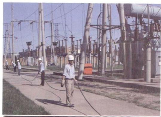
古马220kV变电站施工现场
