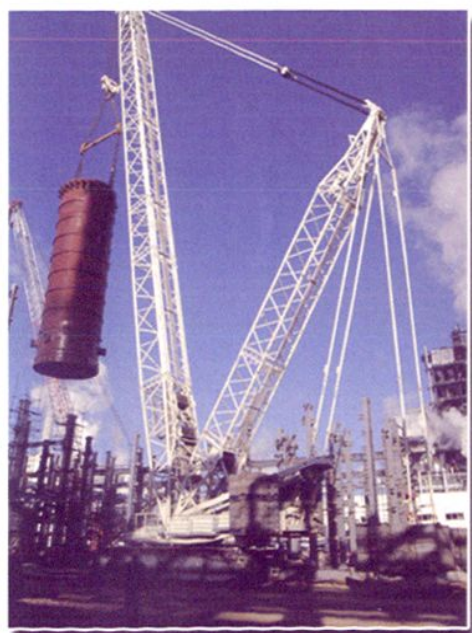
蓝巢吊装承揽的神华829工程项目
