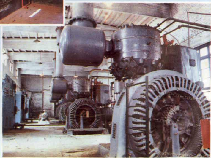
▶ 矿人行井口空气压缩机房
