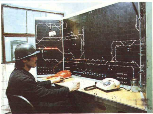
▲ 井下运输信集闭系统
