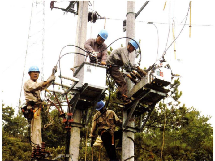
2005 年大田供电所 10 千伏 线路维修
