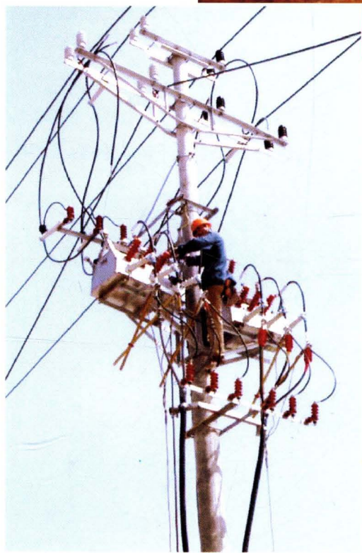
2004 年临海市城区 10 千伏 电力线路环网改造工地
