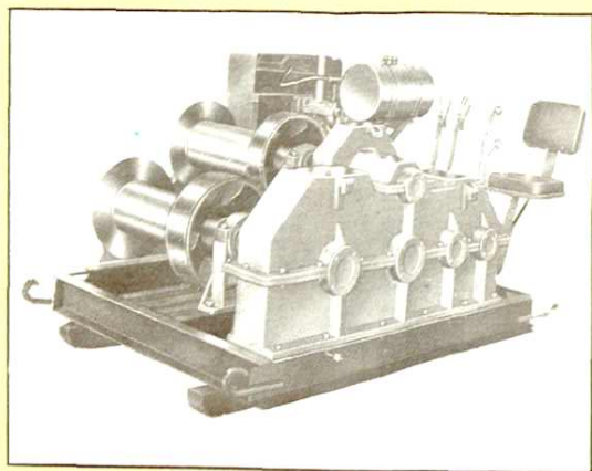
J23A (2-1A) 两筒绞盘机
