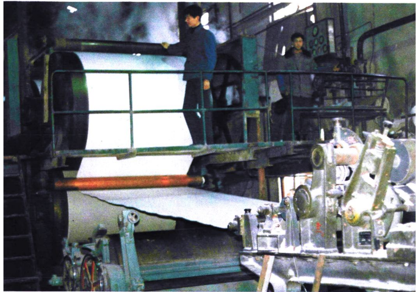
上：汉川县造纸厂造纸车间3号纸机正在生产白板纸。
