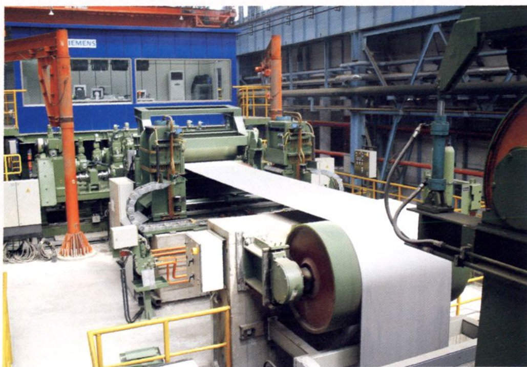
包钢冷轧板生产线
