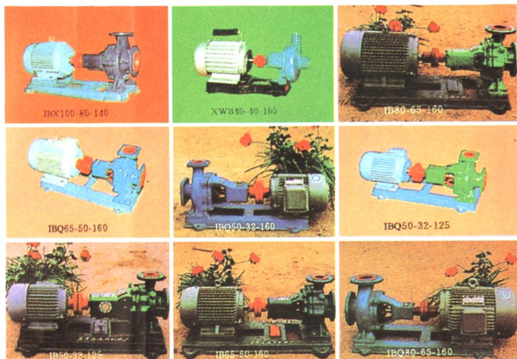
各种型号的高效节能农用水泵
