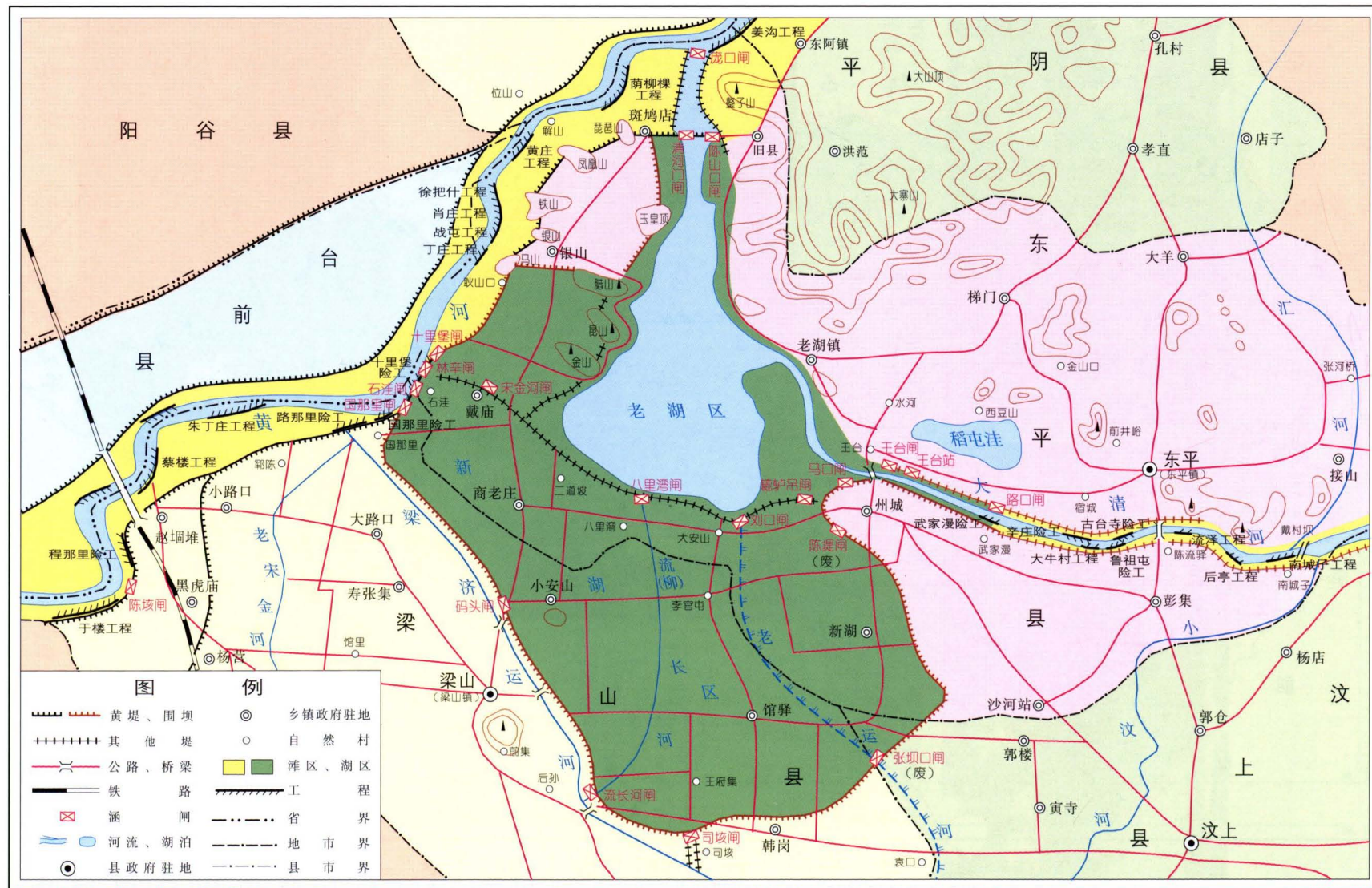
黄河东平湖大清河工程位置图
