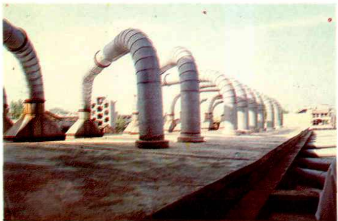
城关棉花加工厂排尘(环保工程)
