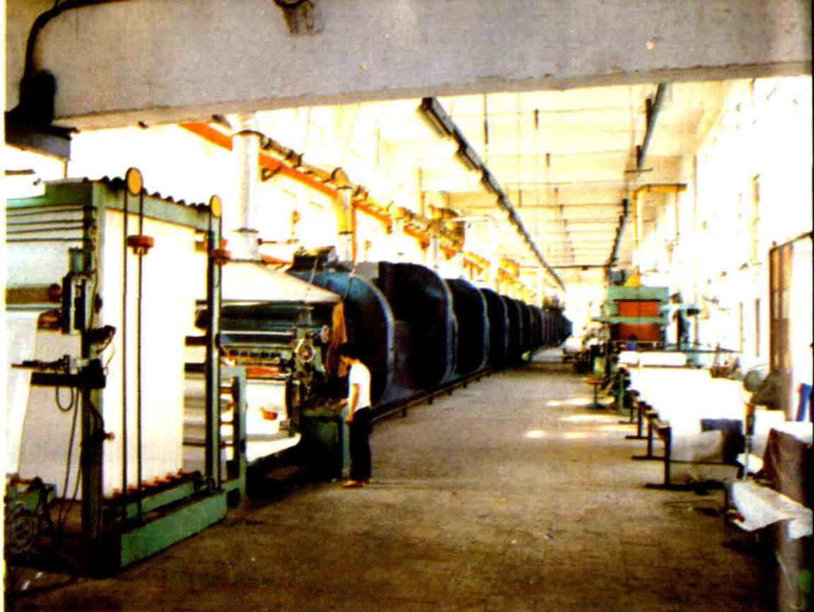
P U 革 生 产 流 水 线
