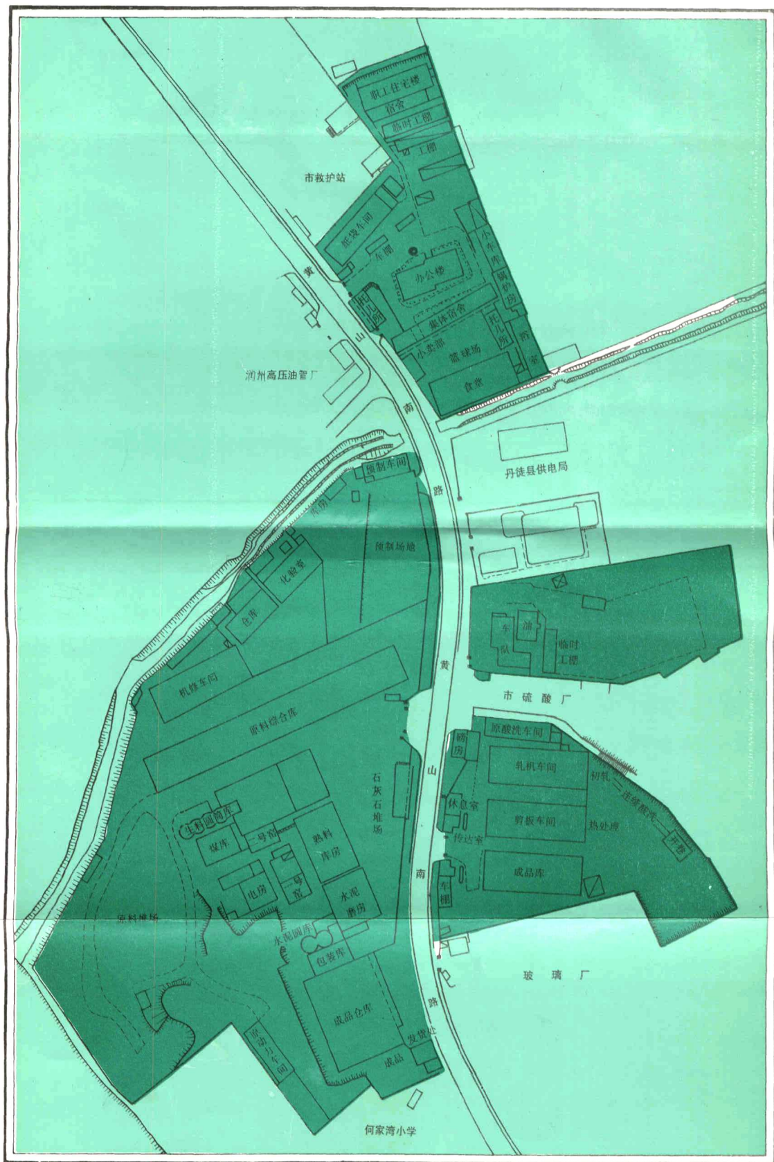
黄山水泥厂平面图
