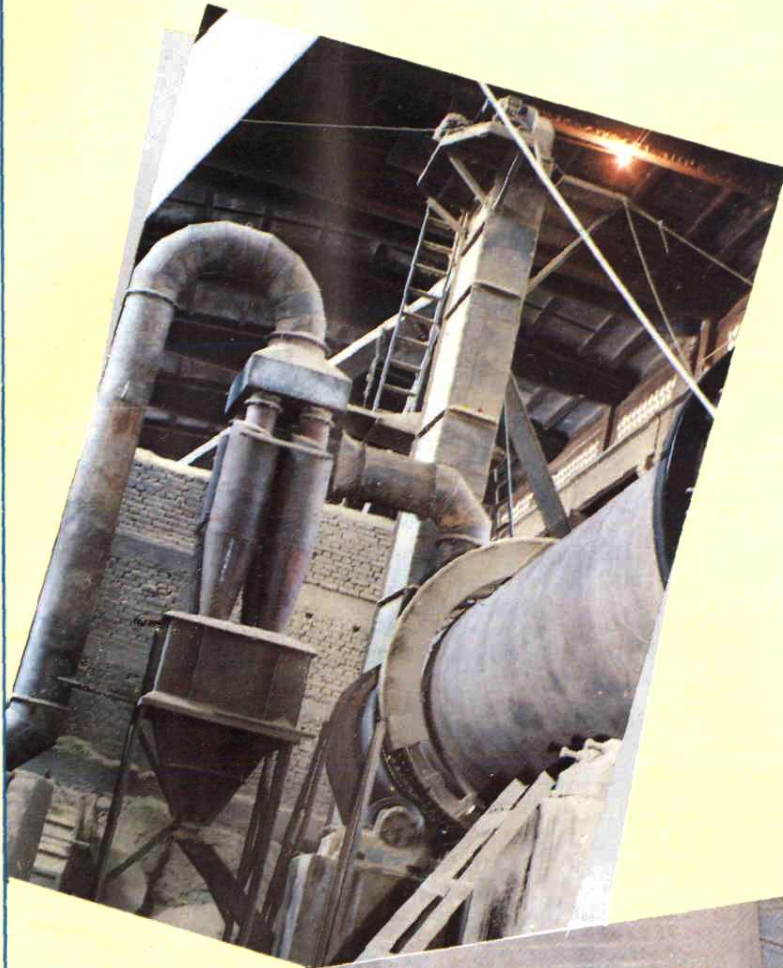
烘干机
