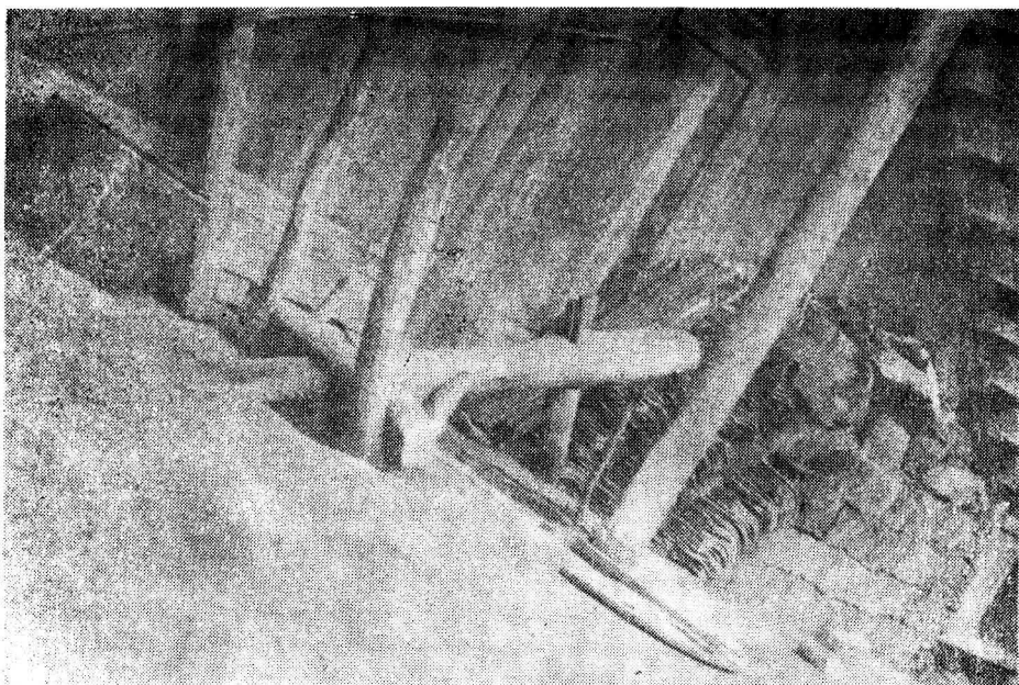
民间脚碓
