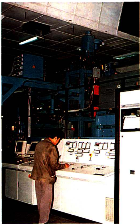
广惠塑胶公司的FFT1600COEX-2型螺杆机生产设备
