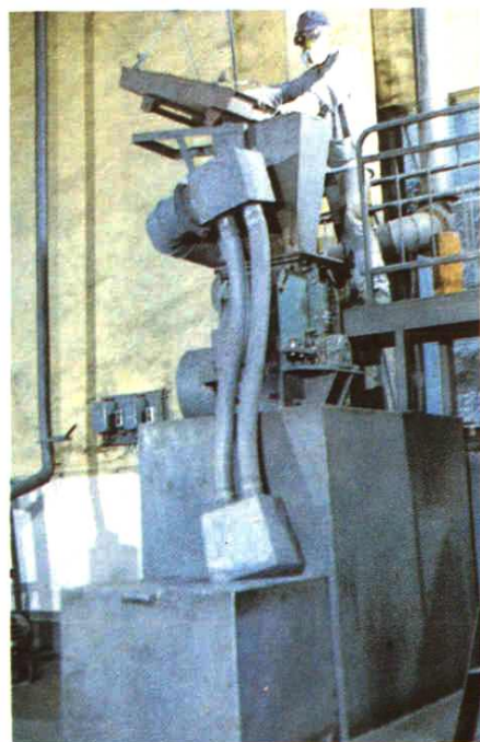
铸造碳化钨破碎机
