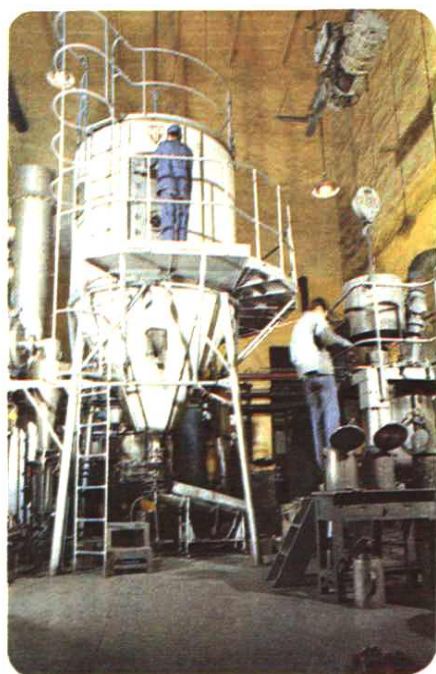
喷雾干燥装置（丹麦引进）
