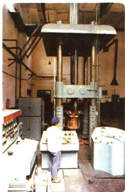
◀ 热压机在工作
