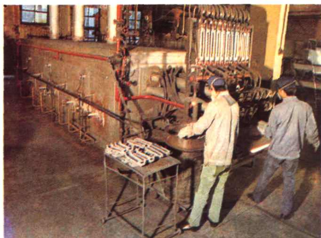
还原炉（制粉车间）
