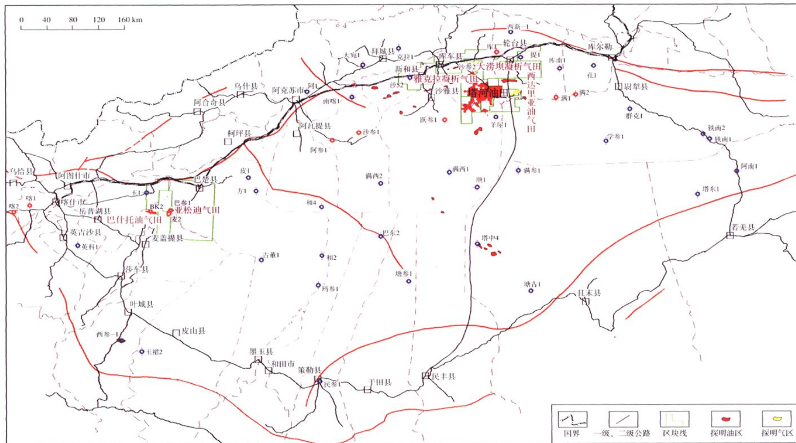
新疆维吾尔自治区塔里木盆地西北油气区油气田分布图
