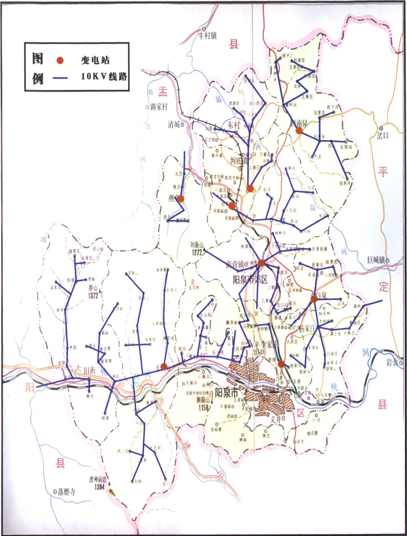
阳泉市郊区10KV线路地理接线示意图
