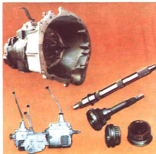
部分汽车变速器总成和零件
