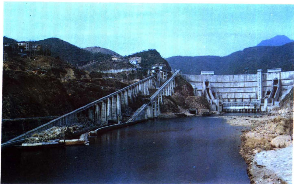
紧水滩水电站坝区船排道(船舶过坝)
