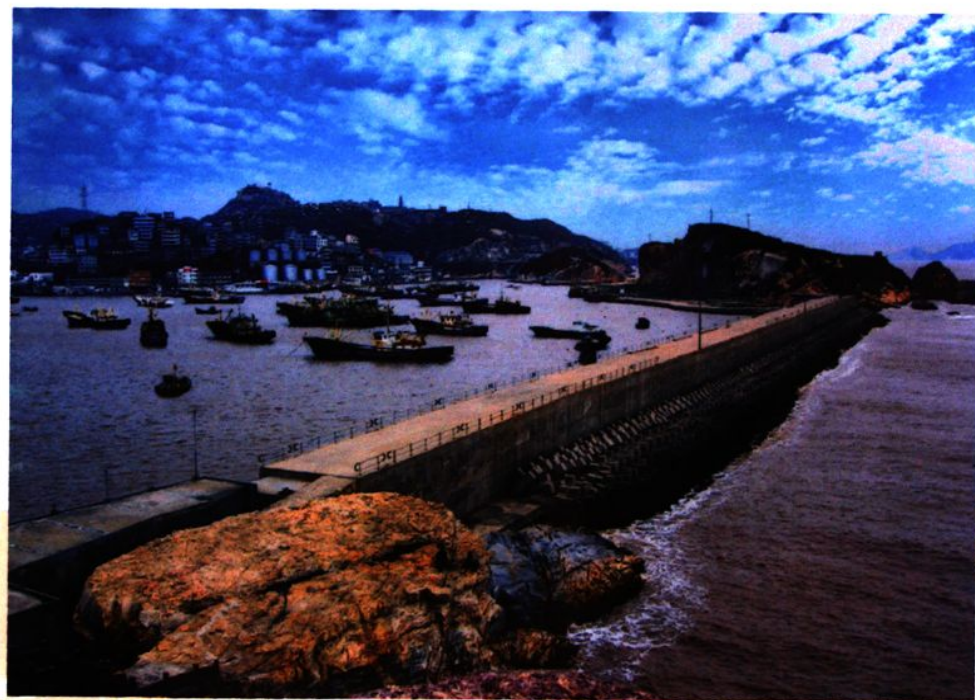
石塘渔港防波堤
