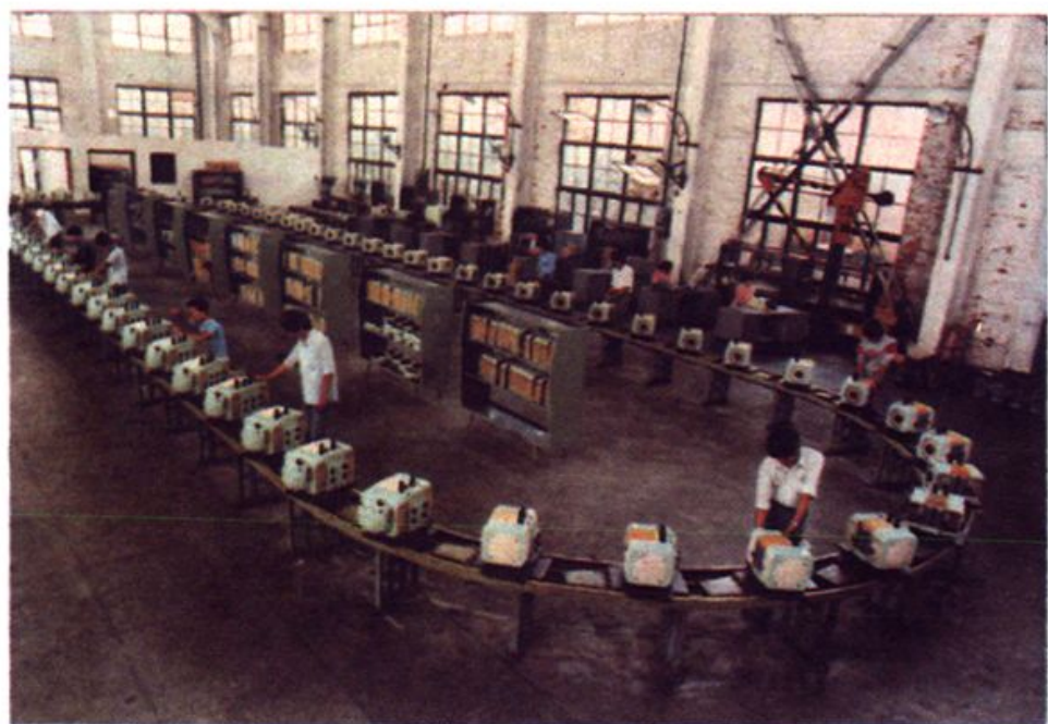
气泵环形装配线
