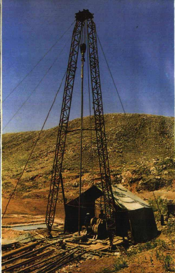
▲ 钻机打井
