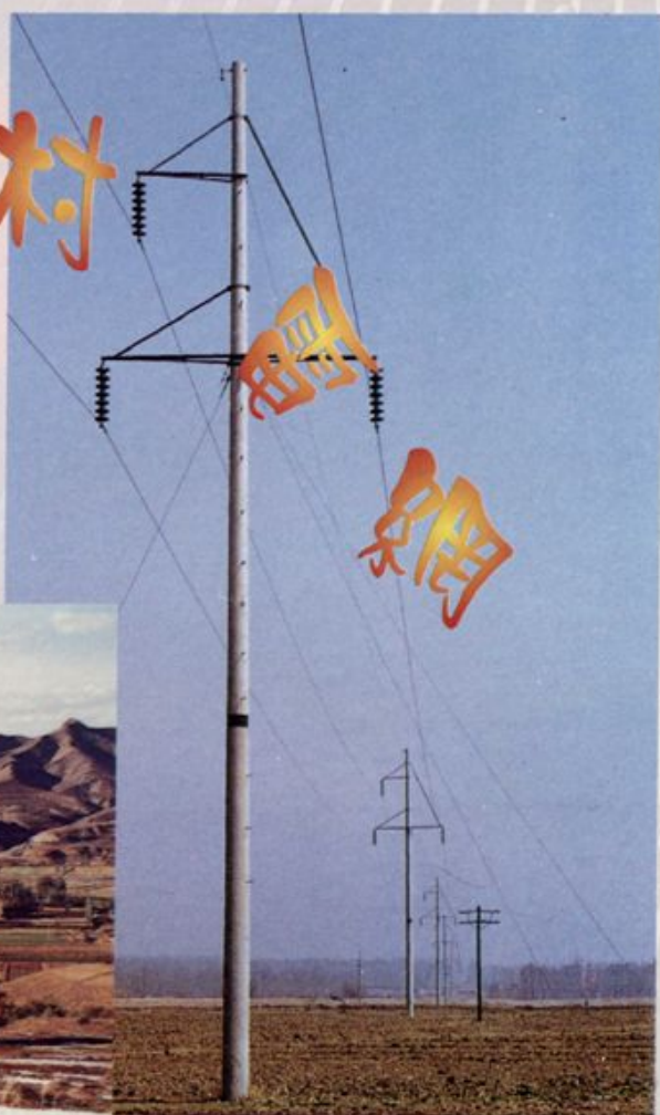
110 千伏送电线路
