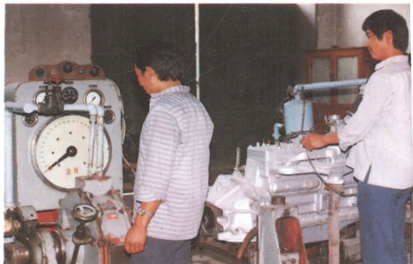
对改造的解放CA-10B型汽车 发动机做台架试验
