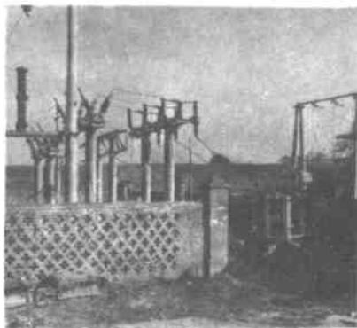
35千伏户外装置
