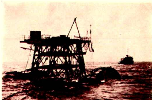
拖航(1964年在莺歌海)
