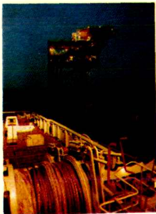
涠10—3油田采油平台在施工中
