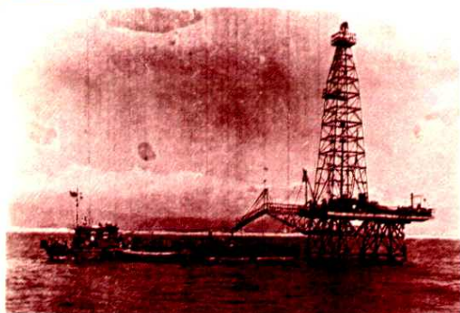
60年代初，我国土法上马，自己制造的第一套海上钻井装置
