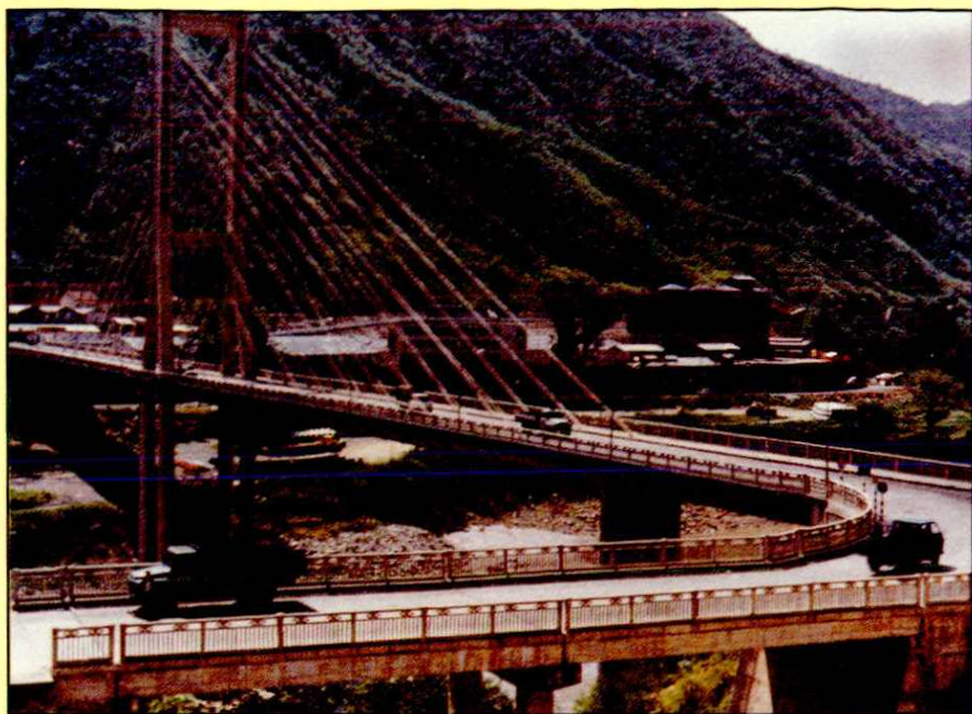
①桐子林单斜拉桥
