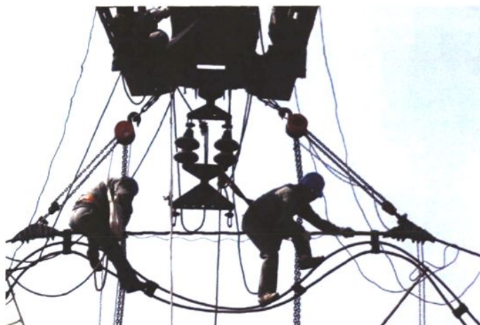
淮南供电公司职工在500千伏高压线路上作业
