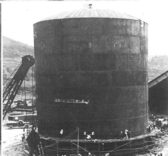
图为安装公司加工厂采用壁板对接充气顶升倒装法分八层拼装 8000m 3 的液氨贮罐正在进行施工收尾。
