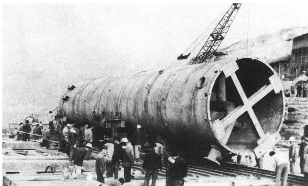
图为安装公司加工厂采用壁板对接充气顶升倒装法分八层拼装 8000m 3 的液氨贮罐正在进行施工收尾。
