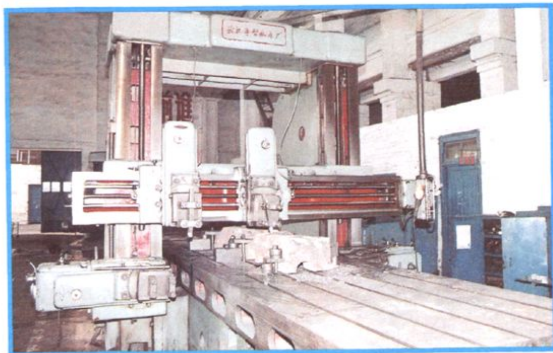
6米龙门刨床
