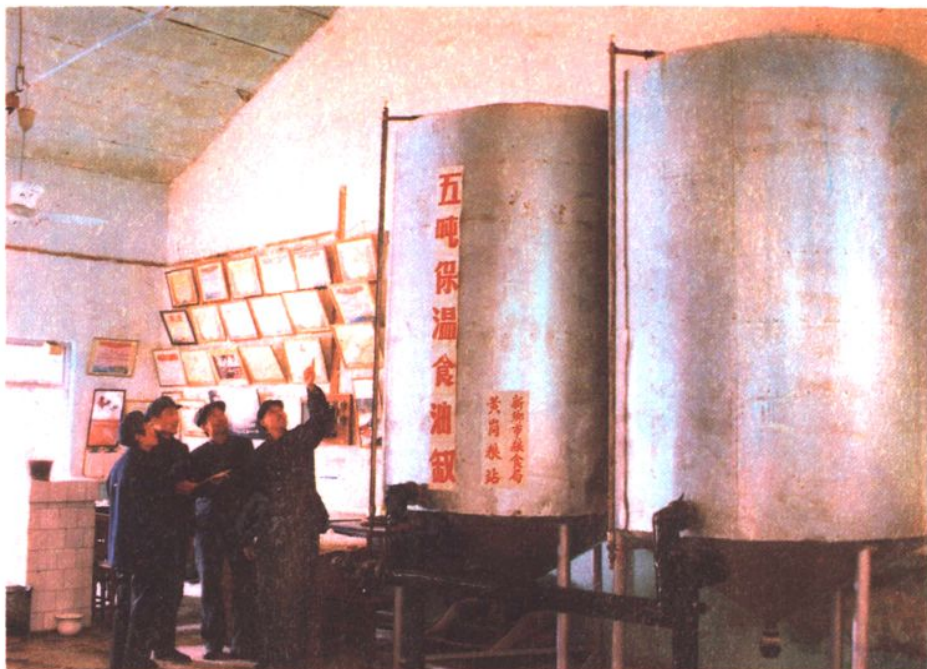
市粮油购销公司一九八五年 为市区粮站设计制造的保温油罐。
