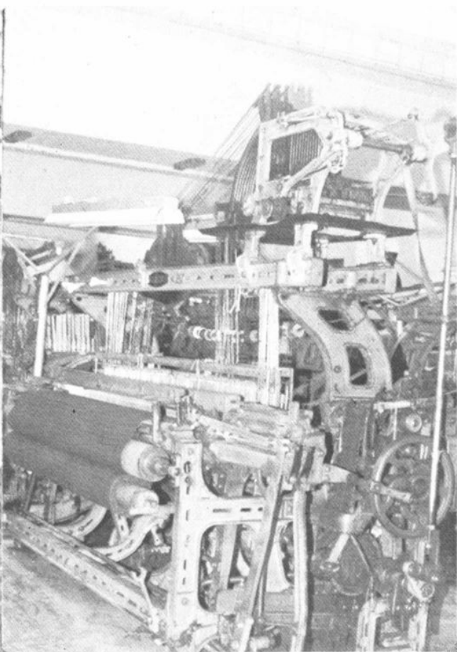
△1515型75" 多臂多梭织机
