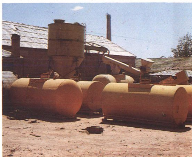
汽车改装二厂生产的Q S型气力式输送机
