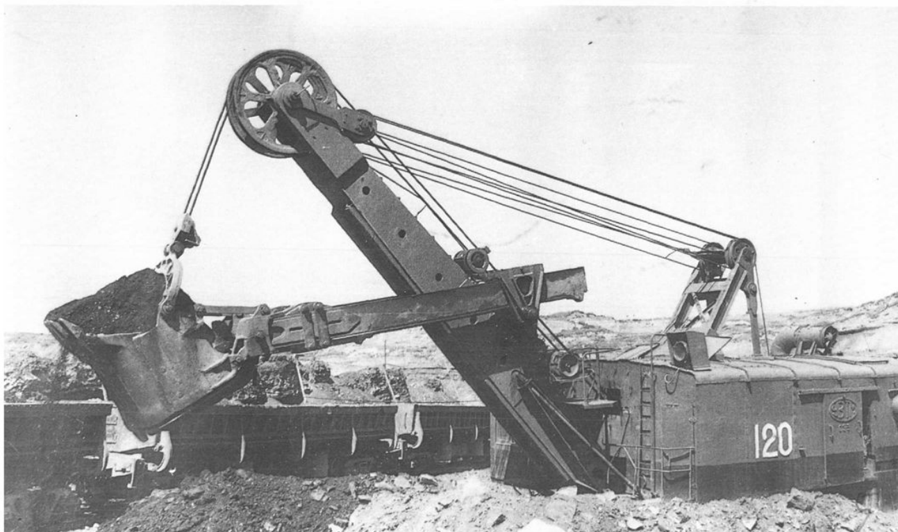
▼露天矿电镐作业现场
