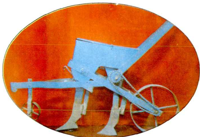
县农机厂生产的山地施肥沟播机
