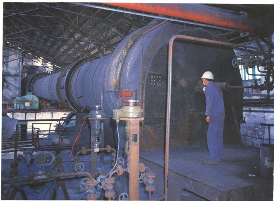
钒铁车间焙烧回转窑
