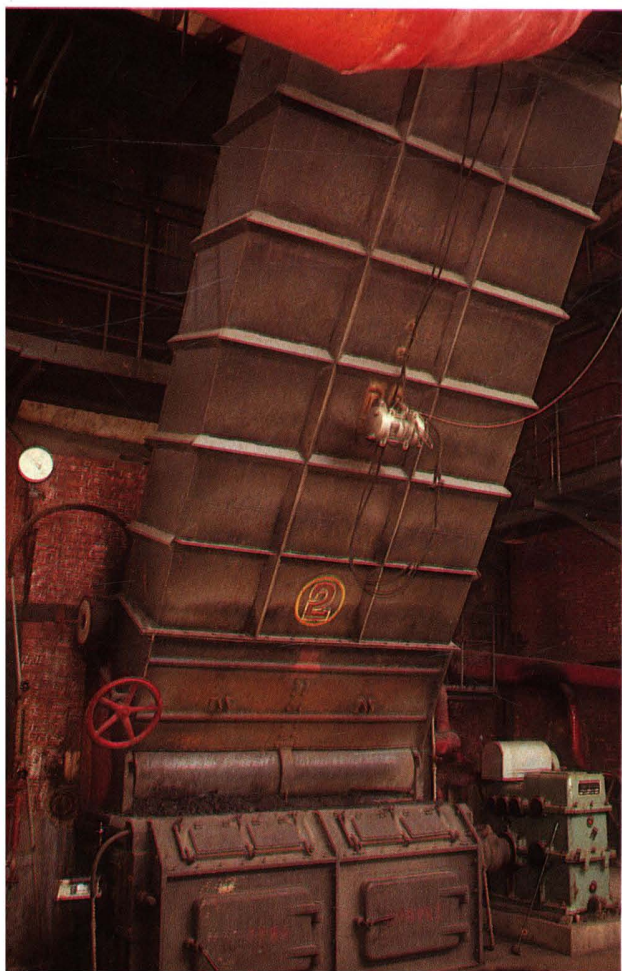
2 號鍋爐
