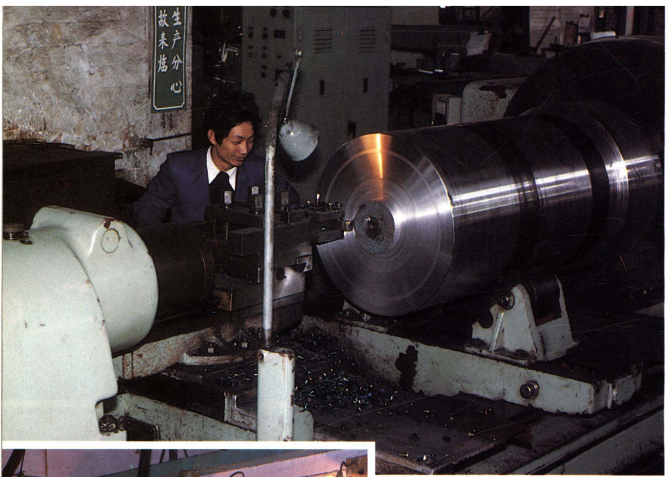
大型鍛件金加工
