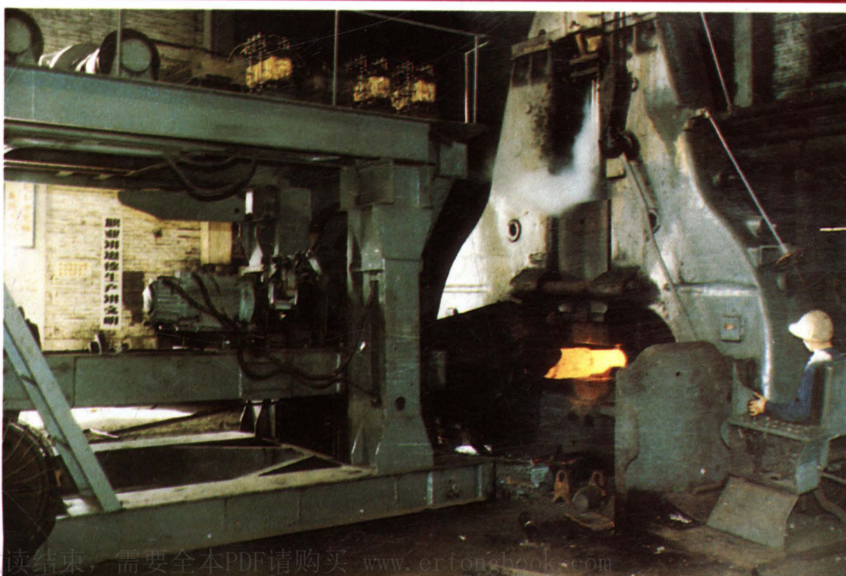
3 噸自由鍛錘在生產
