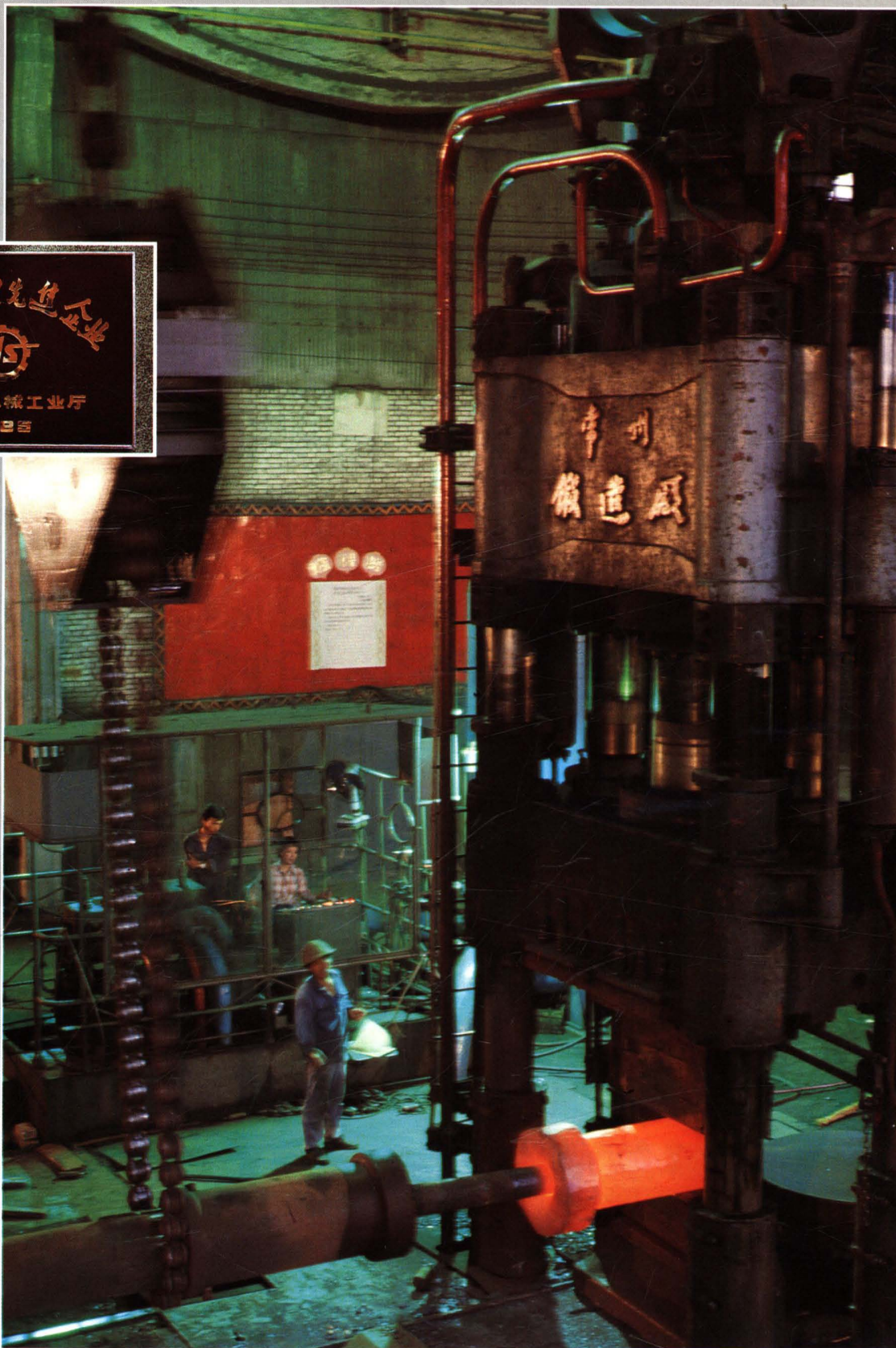
1600噸自由鍛造水壓機在生產
