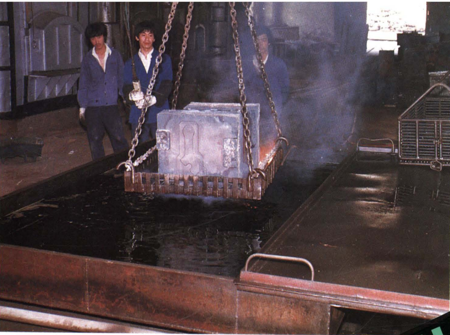
鍛模在熱處理
