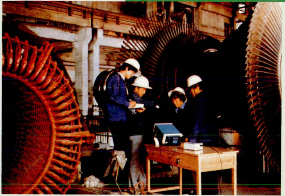
汽轮机叶片超声波探伤
