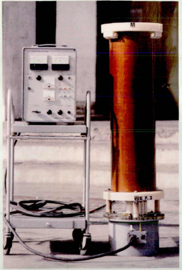
高压试验器——1980年全国电力优质产品
