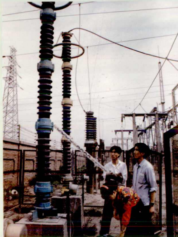
自制 FZ 避雷器带电测试仪
