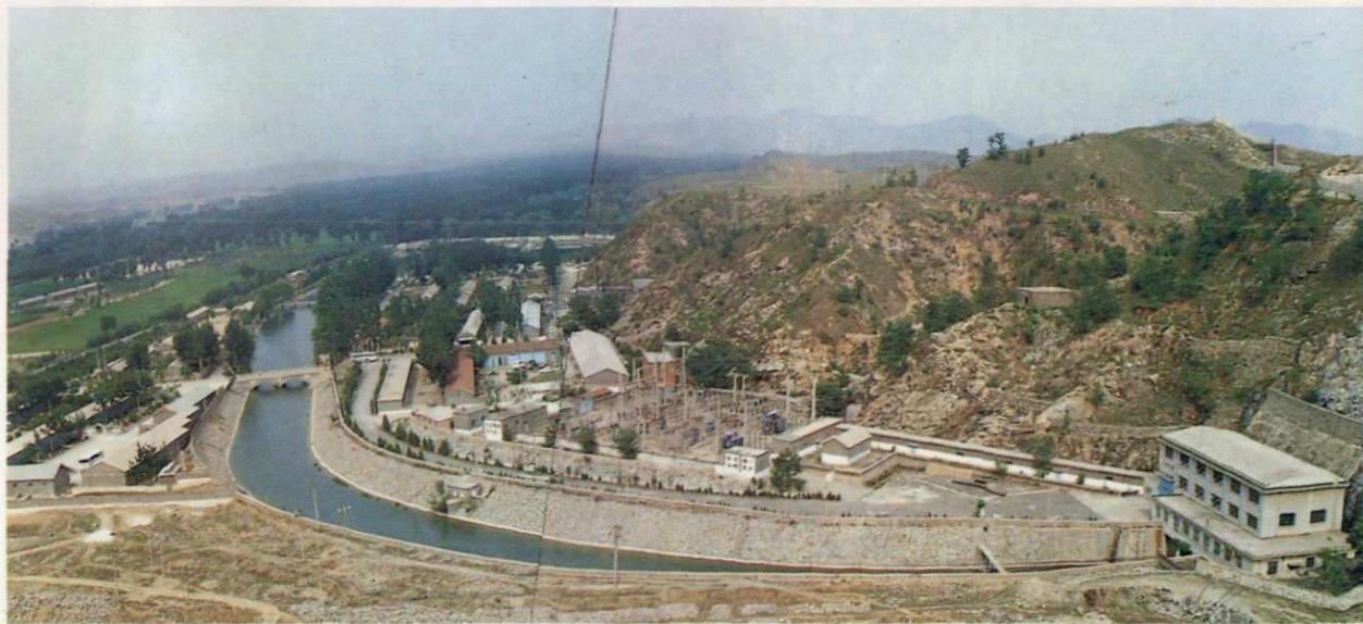
王快水电厂
