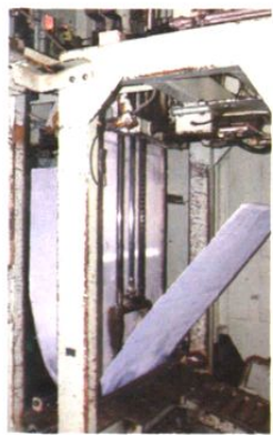
在国内独树一帜的自动剥锌机
