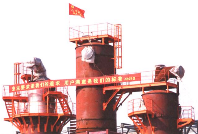
2004年10月的硫酸铅系统干吸
