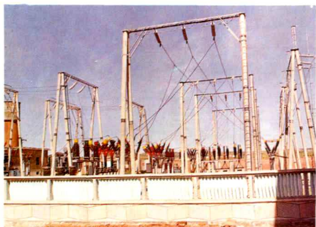
山东黄金总供电所的建成使招掖金矿区的供电日臻完善合理，节能效果显著。图为该所主供电网络及主供电室
