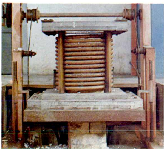
新城金矿的中频电炉
