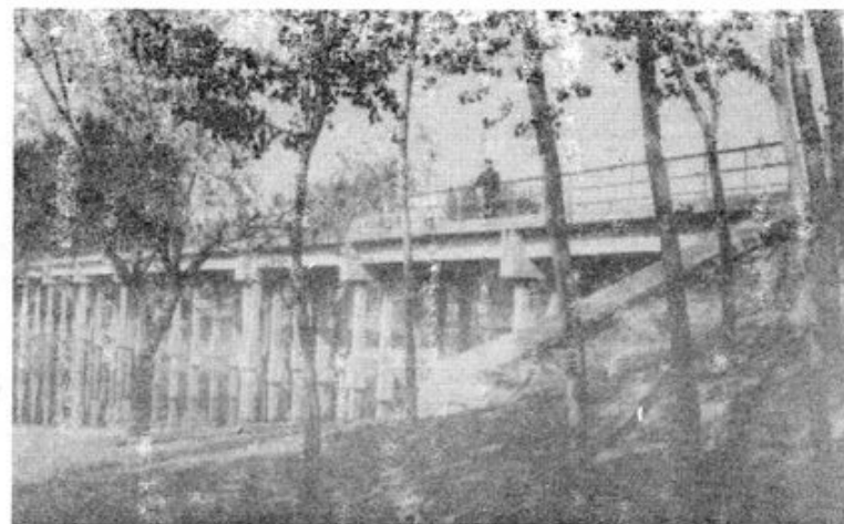
14、徒骇河王把式生产桥
