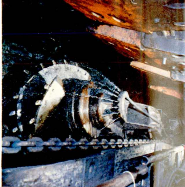
富力煤矿综采工作面
