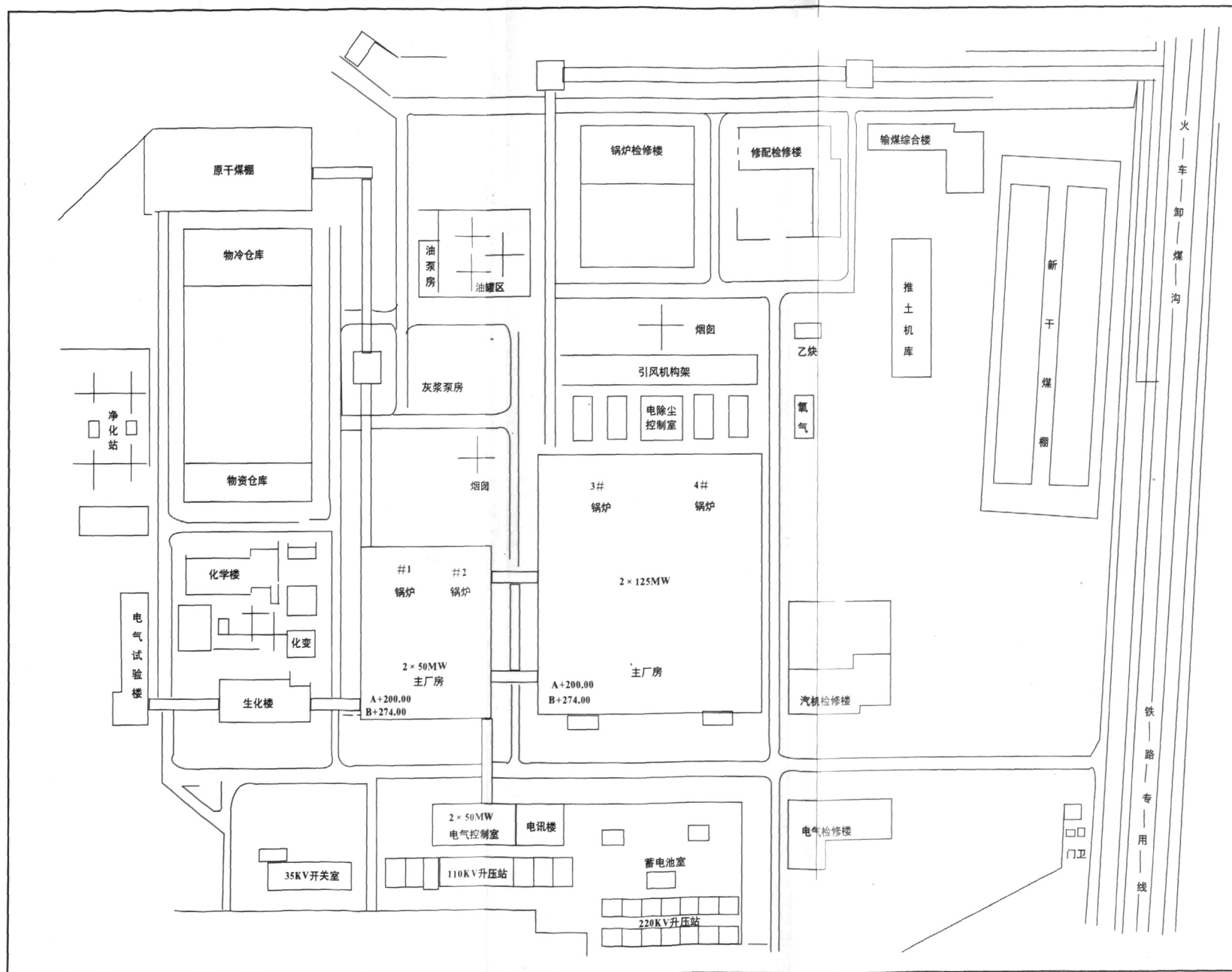
景德镇发电厂技改工程厂区平面布置图
