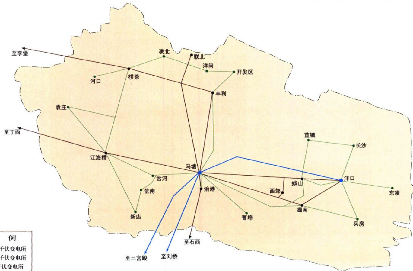
2005年如东电网地理接线示意图
