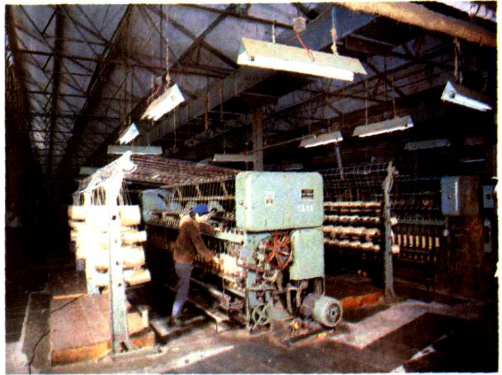
併线
