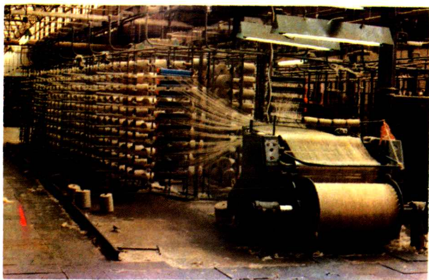
整经
