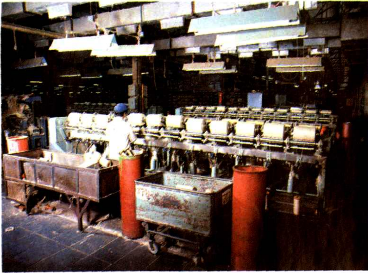
络经
