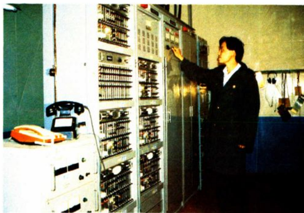
毕节地区邮电局载波电报机房
