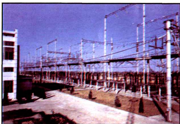
司属安装公司承建的位于南昌市郊的 220 千伏变电站
