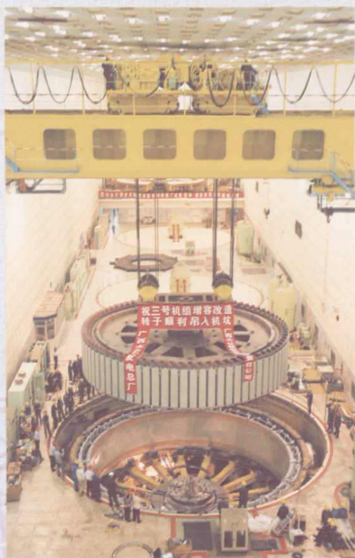
▲ 大化水电厂转子吊装
