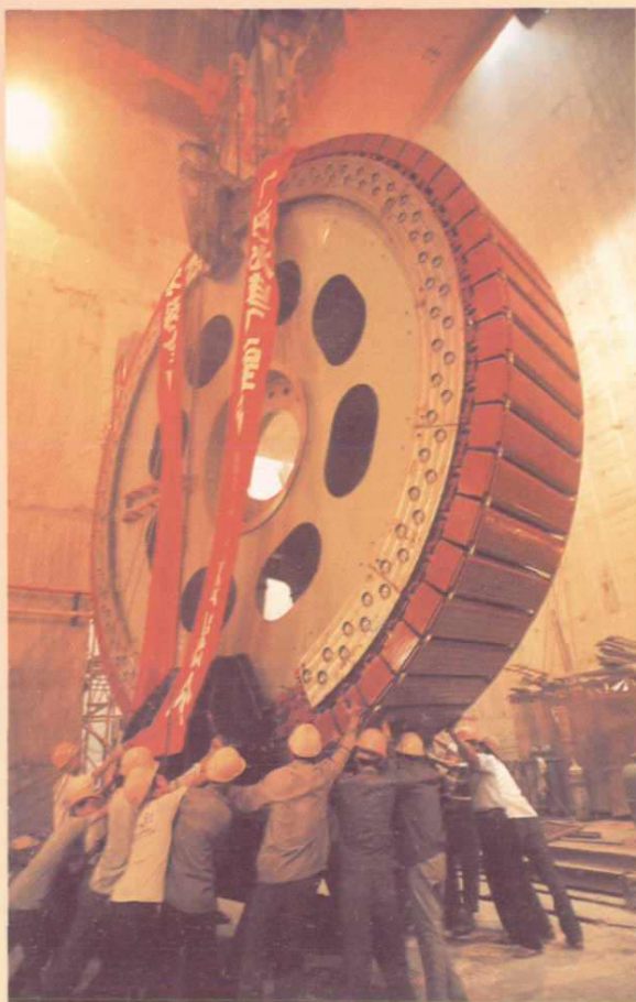
▲ 百龙滩水电厂转子吊装
