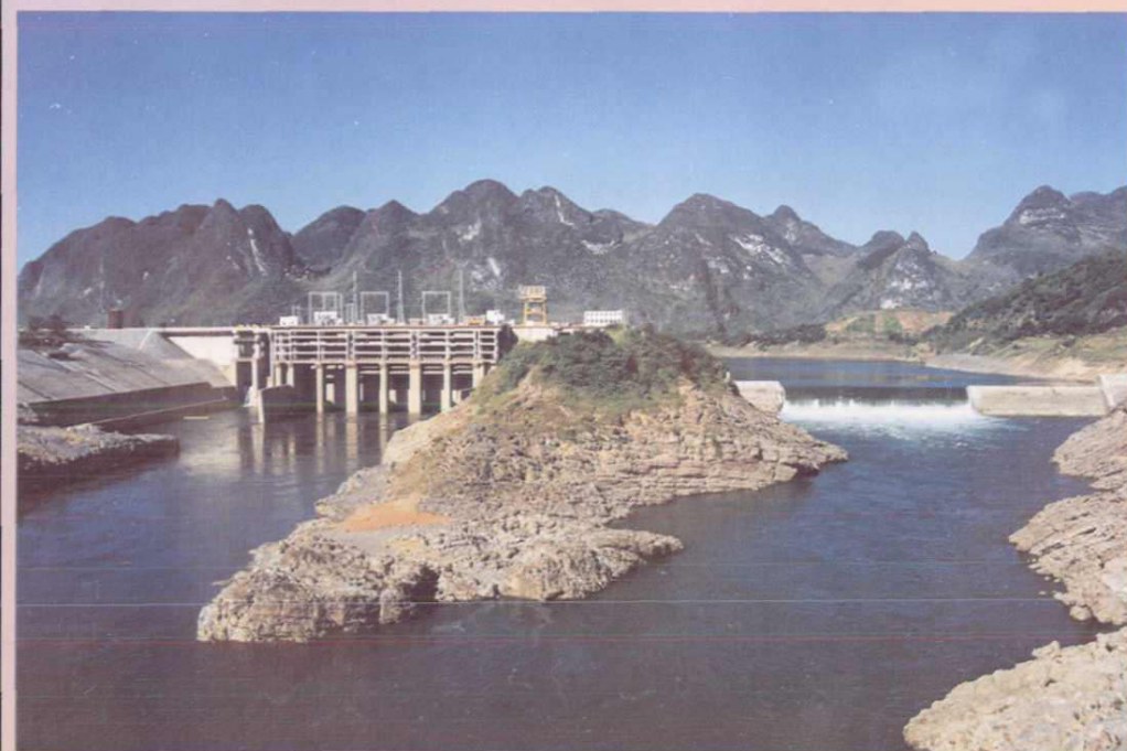
▲ 百龙滩水电厂下游景观
