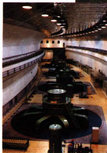
70 年代国内第一座大型空腹重力拱坝——凤滩水电厂全景及其坝内式厂房
