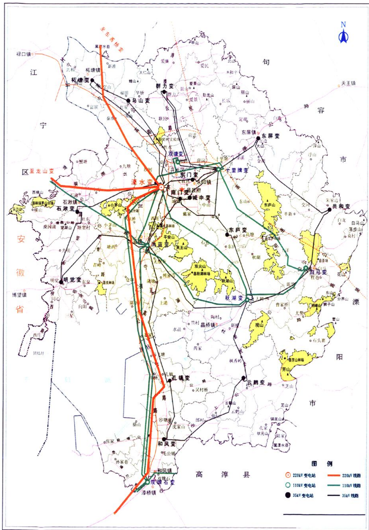
2002年底溧水县35千伏及以上电网地理结线示意图
