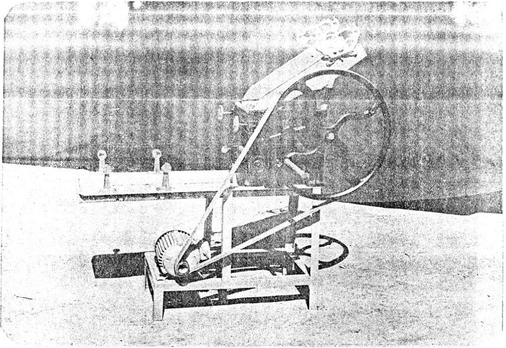
(六) 单头电动压面机
